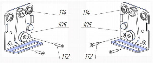
Рис.10.1 Закрепление при установке механизма на ЛЕВОМ щите короба
